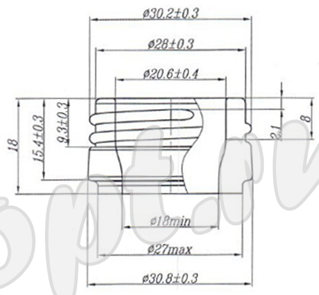
Венчик тип В-31-1 М 2:1
