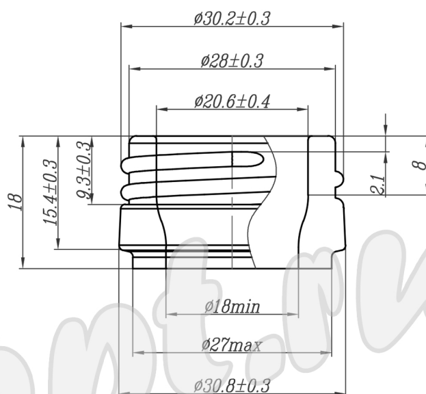
Венчик тип В-31-1 М 2:1
